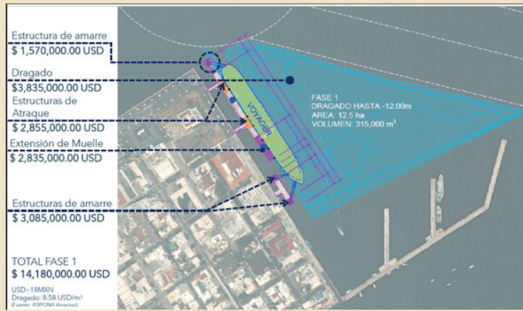
MUELLE TURÍSTICO DE CRUCEROS (LICITACIÓN)
